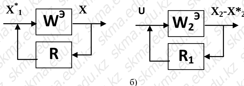
Сурет 9.5 – (а) – негізгі және (б) қосымша реттегішті эквивалентті бірконтурлы АРЖ құрылымдық схемасы
